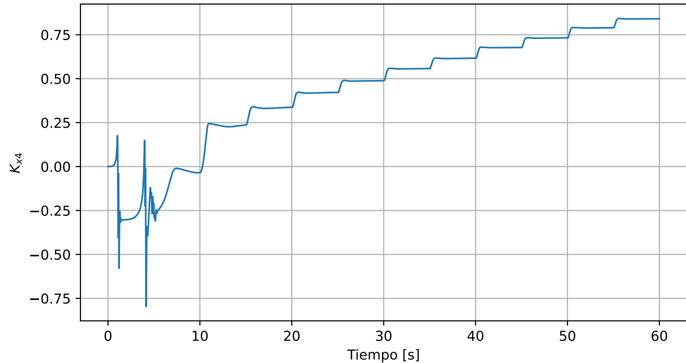
Evolución de K_{x4} - tren de pulsos
